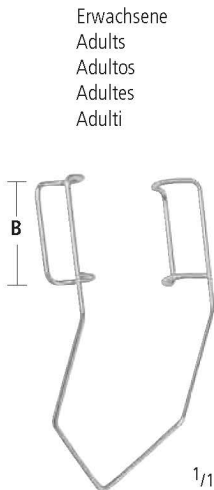
BARRAQUER-COLIBRI B 15 mm KP 150/15 4,0 cm/1½"
